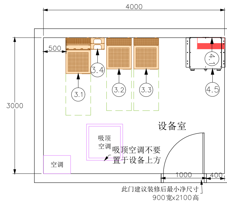
系统布局图
